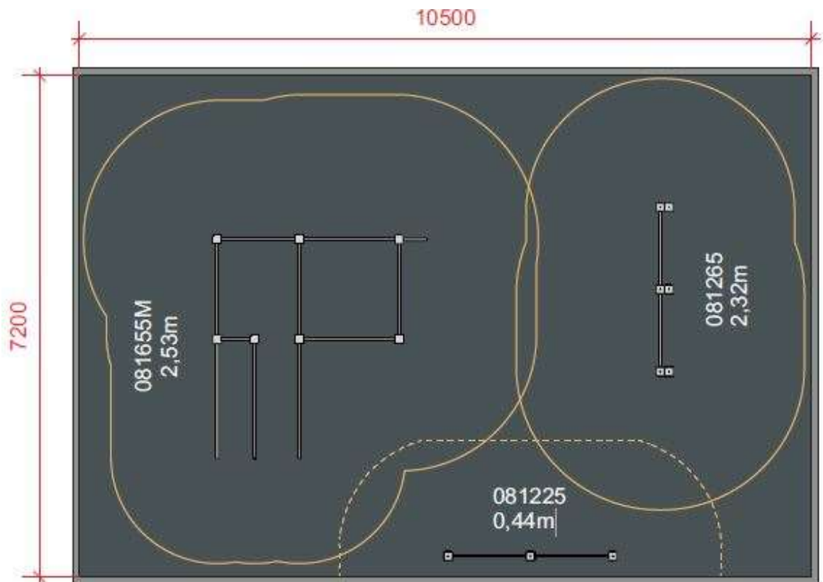
Inrichtingstekening sportplek: links het calisthenics toestel, rechts de hoge bar en aan de onderkant opdruksporten
