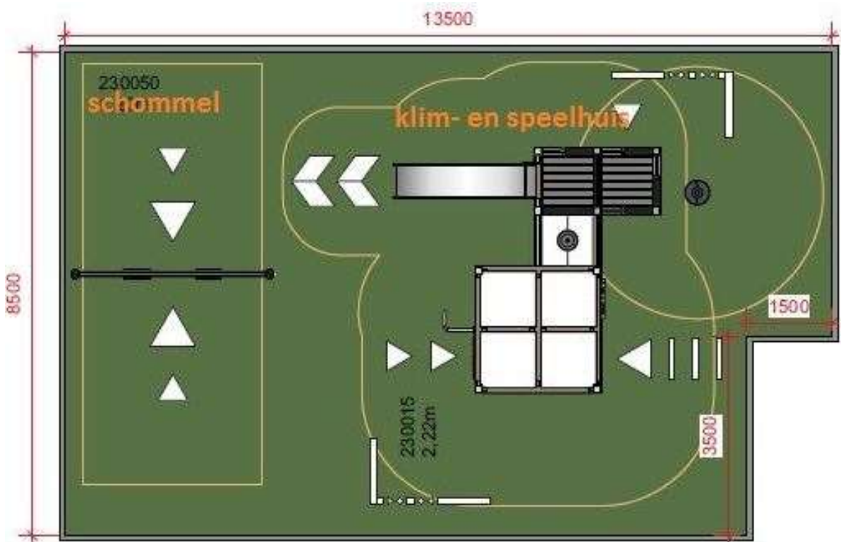
Inrichtingstekening speelplek: links de schommel en rechts het klimhuis
